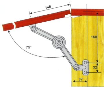
75° 安装尺寸图 Installation sizes
