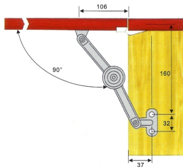
90° 安装尺寸图 Installation sizes
