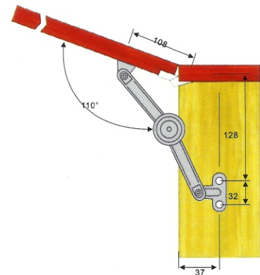
110° 安装尺寸图 Installation sizes
